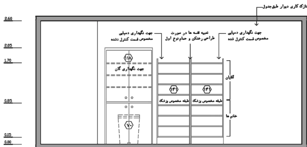
نما ۱ - مقیاس : ۱:۵۰
