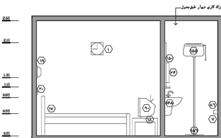
نما ۳ - مقیاس : ۱:۵۰
