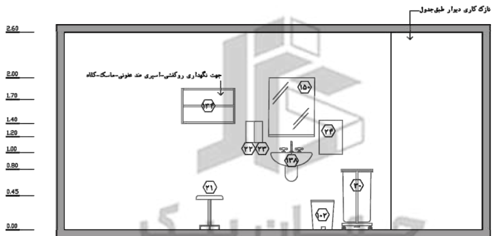
نما ۲ - مقیاس : ۱:۵۰
