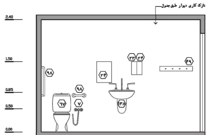
نما ۶- مقیاس : ۱:۵۰
