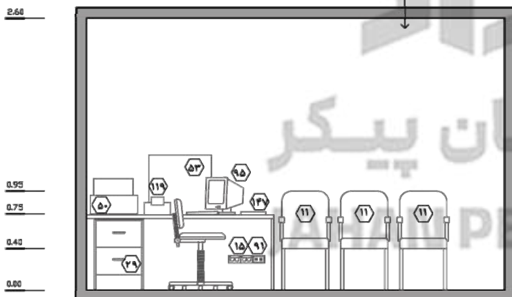
نما ۱ - مقیاس : ۱:۵۰
