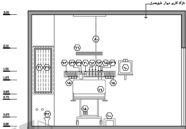
نما ۲- مقیاس : ۱:۵۰
