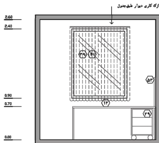
نما ۴ - مقیاس : ۱:۵۰
