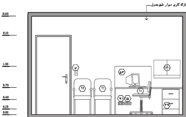
نما ۱ - مقیاس : ۱:۵۰
