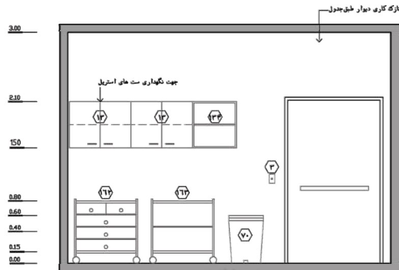
نما ۲- مقیاس: ۱:۵۰
