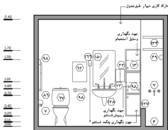
نقشه ۲-۱۴ - نما ۱ - مقیاس ۱:۵۰
