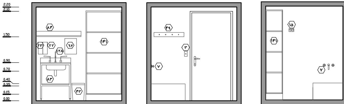
نقشه ۵۹-۲- نما ۱- مقیاس ۱:۵۰
