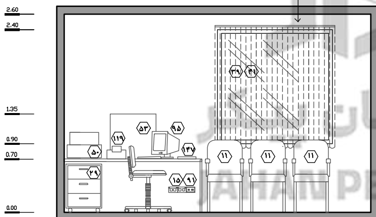
نقشه ۲-۴۴- نما ۱- مقیاس ۱:۵۰
