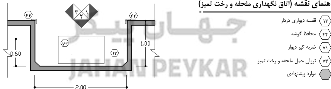
نقشه ۲-۷۰- پلان فضا/اتاق نگهداری ملحفه و رخت تمیز - مقیاس ۱:۵۰
