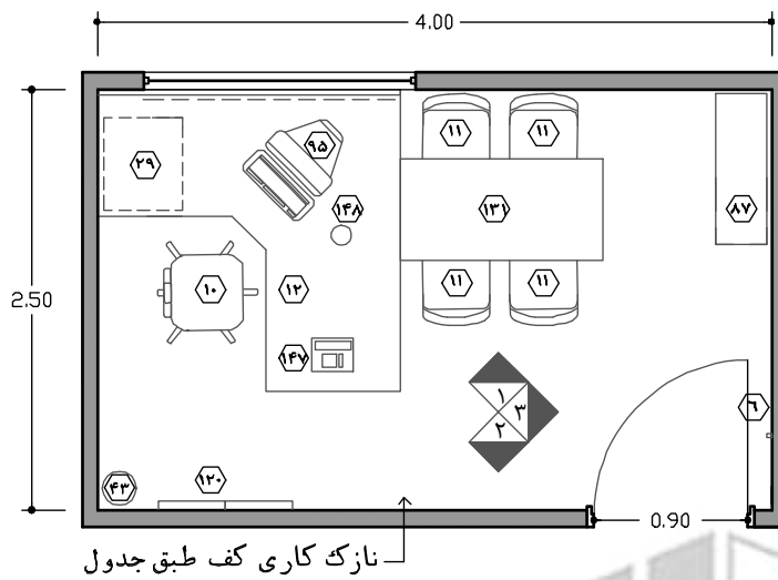
نقشه ۲-۴۷- پلان دفتر کار سرپرستار بخش - مقیاس ۱:۵۰
