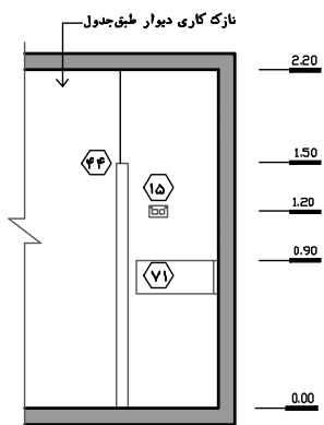
نقشه ۲-۲-۲۲- نما ۲- مقیاس ۱:۵۰
