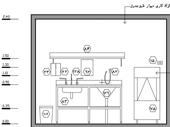
نقشه ۵۶-۲- نما ۱- مقیاس ۱:۵۰
