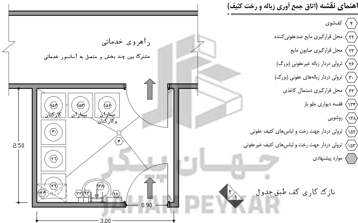
نقشه ۲-۶۲- پلان اتاق جمع‌آوری زباله و رخت کثیف- مقیاس ۱:۵۰
