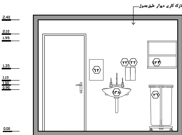
نقشه ۲-۶۳- نما ۱- مقیاس ۱:۵۰
