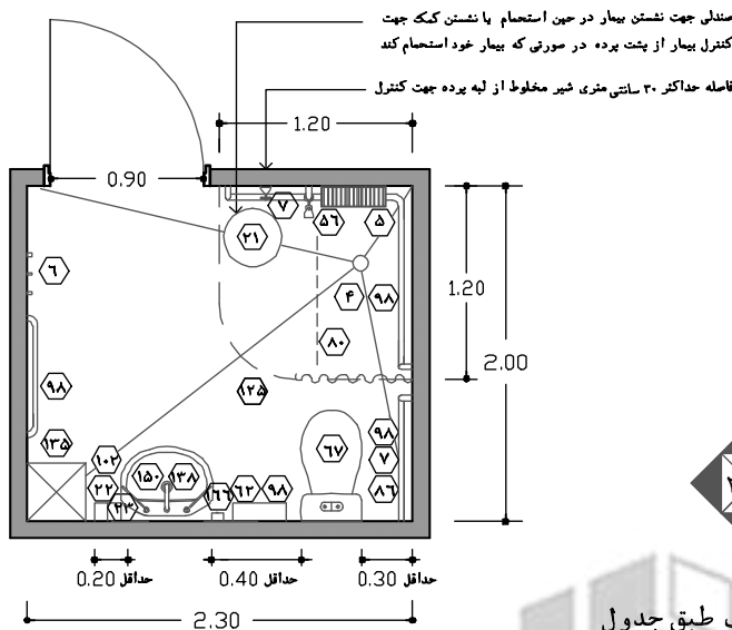
نقشه ۲-۸- پلان حمام و سرویس بهداشتی با امکان ورود ویلچر- مقیاس ۱:۵۰
