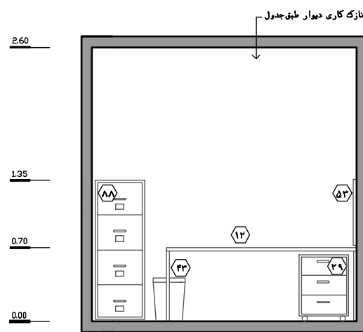
نقشه ۲-۴۶- نما ۳- مقیاس ۱:۵۰
