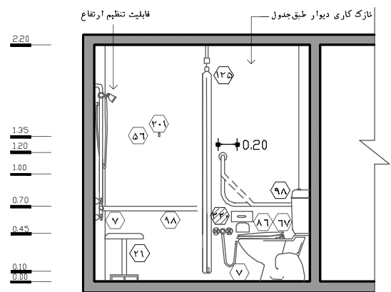
نقشه ۲-۲۱ - نما ۲ - مقیاس ۱:۵۰
