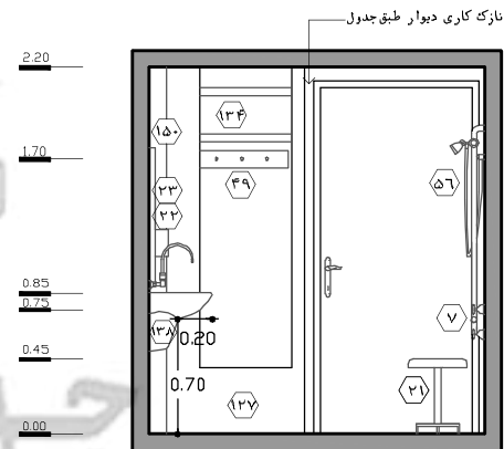
نقشه ۲-۲۳ - نما ۴ - مقیاس ۱:۵۰
