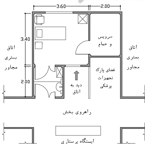
نقشه ۱۸-۲- روش دوم چیدمان اتاق بستری ایزوله در بخش مقیاس ۱:۱۵۰
