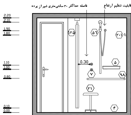
نقشه ۱۰-۲ - پلان اتاق بستری دو تخت خوابی مقیاس ۱:۵۰
