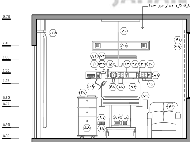
نقشه ۲-۲۴ - نما ۵ - مقیاس ۱:۵۰
