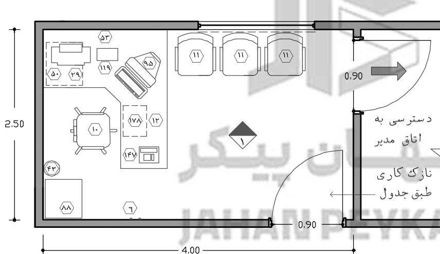
نقشه ۲-۵۳- اتاق منشی اداری - مقیاس ۱:۵۰
