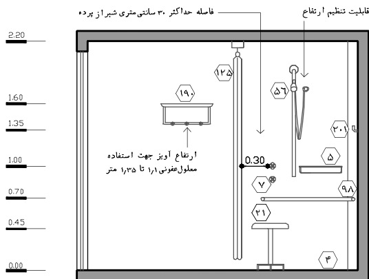
نقشه ۲-۲۰ - نما ۱ - مقیاس ۱:۵۰
