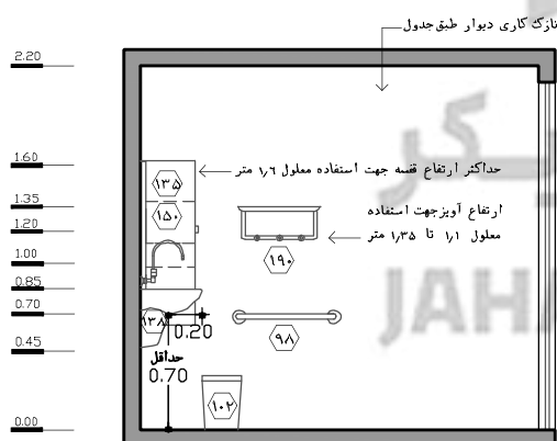
نقشه ۲-۹۳- نمای ۱ - مقیاس ۱:۵۰
