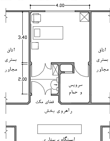
نقشه ۱۷-۲- روش اول چیدمان اتاق بستری ایزوله در بخش مقیاس ۱:۱۵۰
