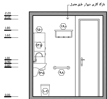
نقشه ۱۲-۲ - نما ۱ - مقیاس ۱:۵۰
