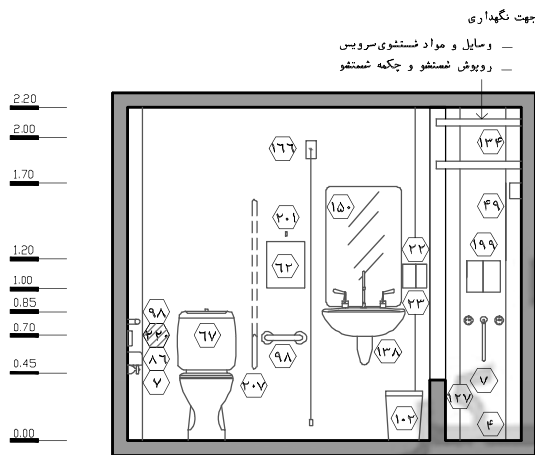
نقشه ۲-۲۲ - نما ۳ - مقیاس ۱:۵۰
