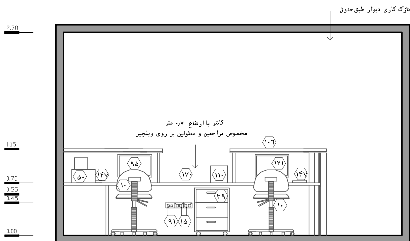
نقشه ۳-۲-۳۱ - نما ۱ - مقیاس ۱:۵۰
