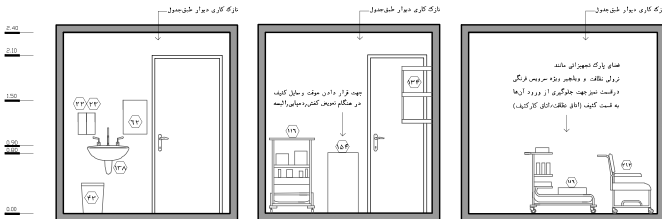
نقشه ۲-۵۸- نما ۱ - مقیاس ۱:۵۰
