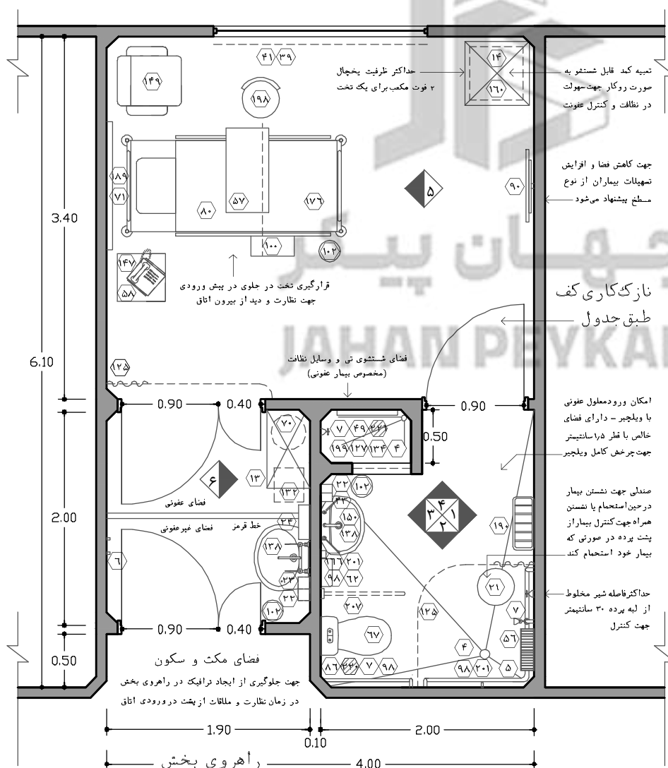
نقشه ۱۹-۲- پلان اتاق بستری ایزوله - مقیاس ۱:۵۰
