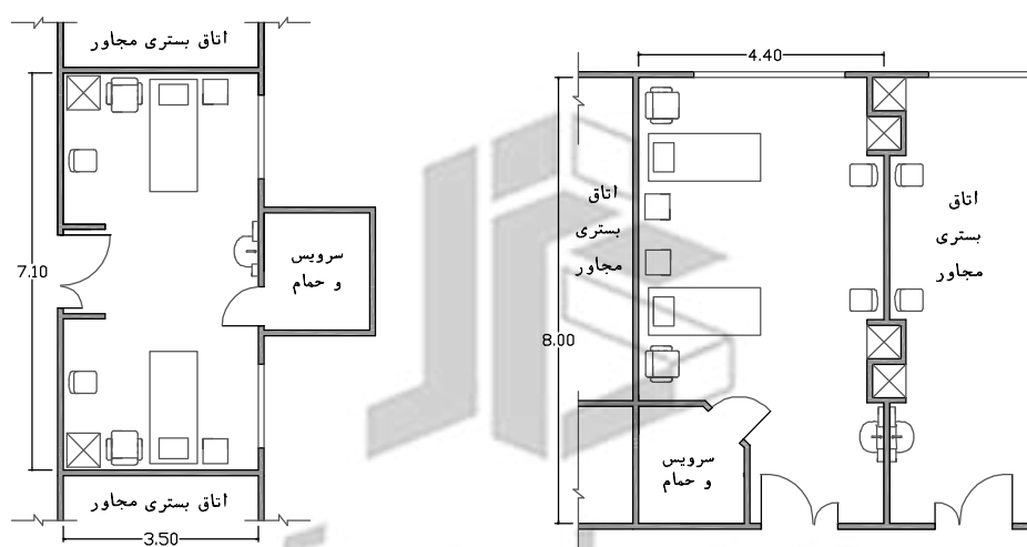
نقشه ۲-۹- روش دوم چیدمان اتاق بستری دو تخت خوابی مقیاس ۱:۱۵۰
