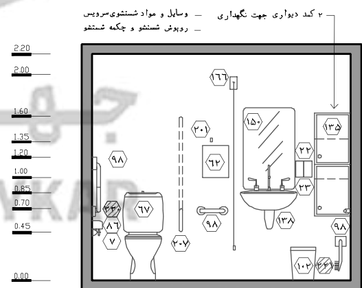
نقشه ۲-۹۴- نمای ۲ - مقیاس ۱:۵۰
