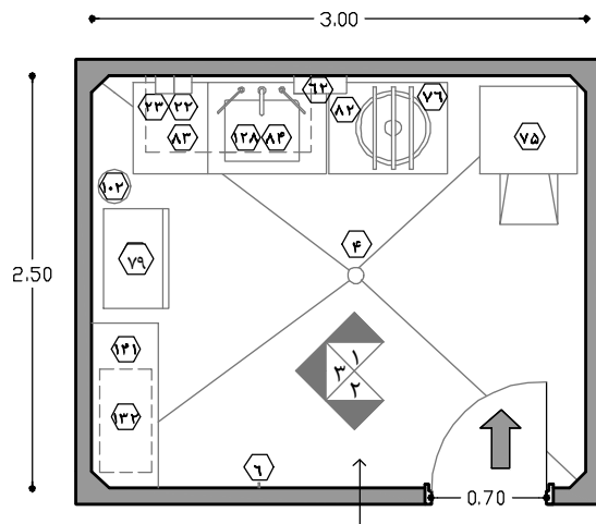
نقشه‌ی ۲-۹۴- پلان نمونه‌ی اتاق کار کثیف (برای ۴۰۰۰ زایمان سالیانه) - مقیاس ۱:۵۰
