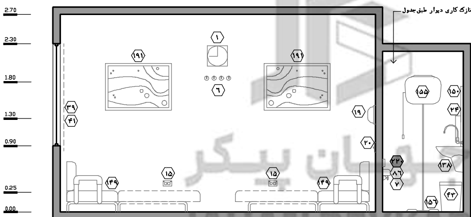
نقشه‌ی ۲-۸۷- نمای ۲ - مقیاس ۱:۵۰
