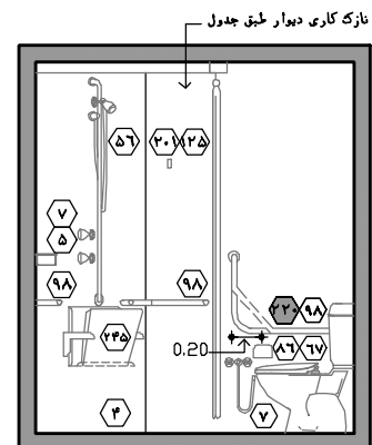
نقشه ۵-۳۹-۲ - نمای ۵ - مقیاس ۱:۵۰
