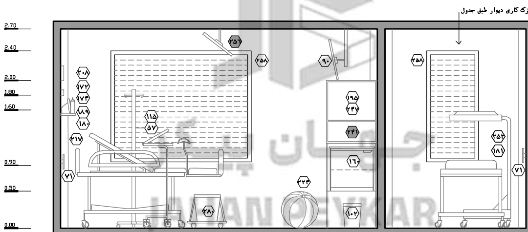
نقشه‌ی ۶۱-۲- نمای ۱ - مقیاس ۱:۵۰
