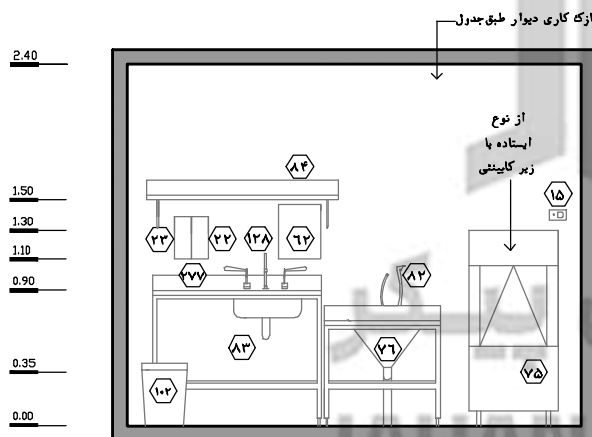
نقشه‌ی ۲-۹۵- نمای ۱ - مقیاس ۱:۵۰
