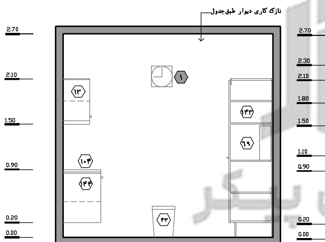
نقشه ۲-۷۷ - نمای ۳ - مقیاس ۱:۵۰
