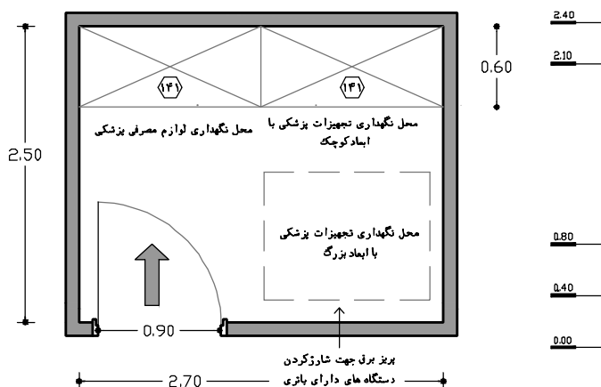
نقشه‌ی ۲-۱۱۷- پلان انبار تجهیزات پزشکی و وسایل مصرفی (برای ۴۰۰۰ زایمان سالیانه) - مقیاس ۱:۵۰
