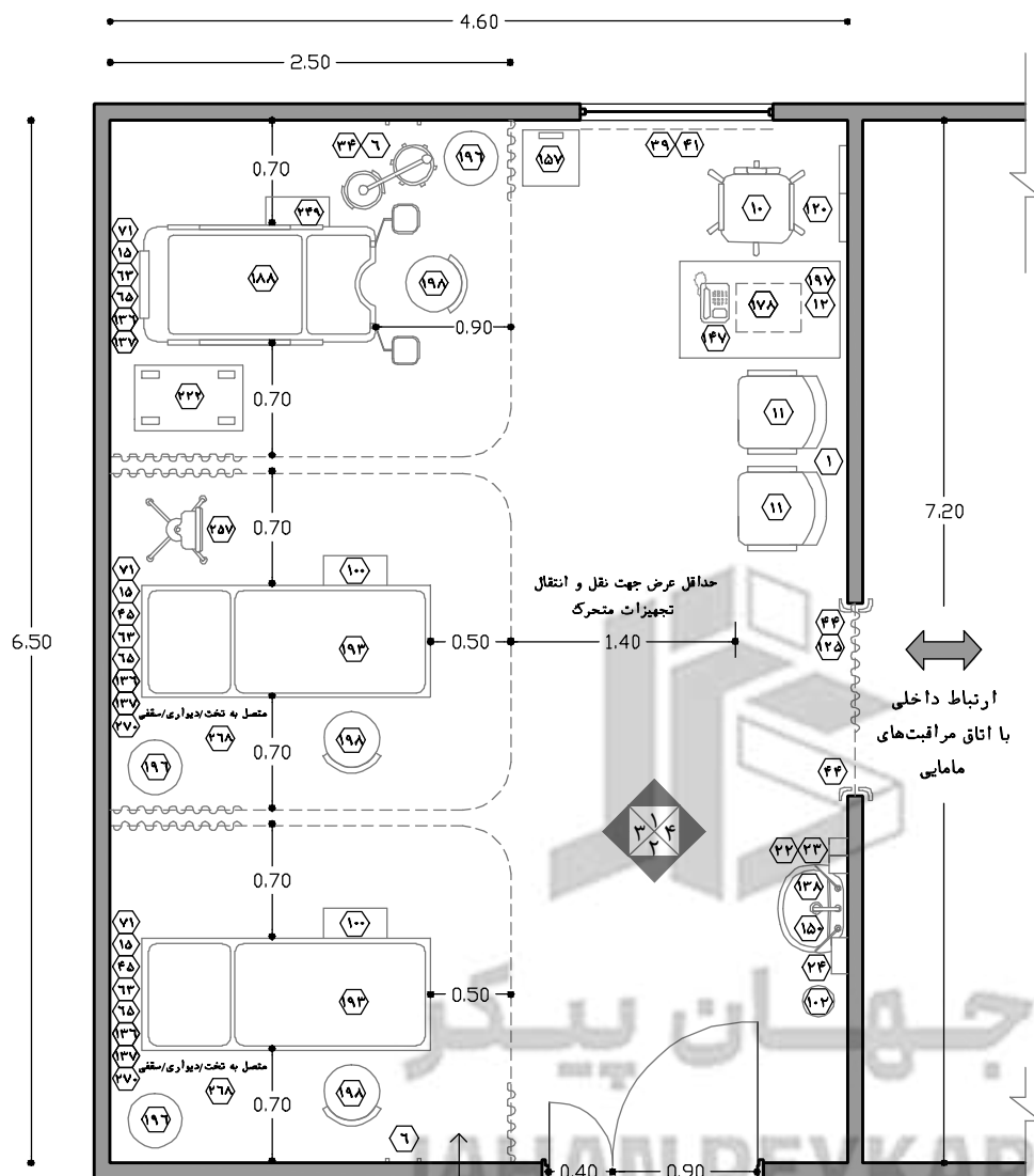
نقشه‌ی ۲-۱۶- پلان نمونه‌ی اتاق معاینه (۴۰۰۰ زایمان سالیانه) مقیاس ۱:۵۰
