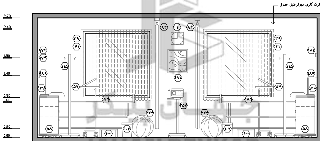
نقشه ۲-۴۲-نمای ۲ - مقیاس ۱:۵۰
