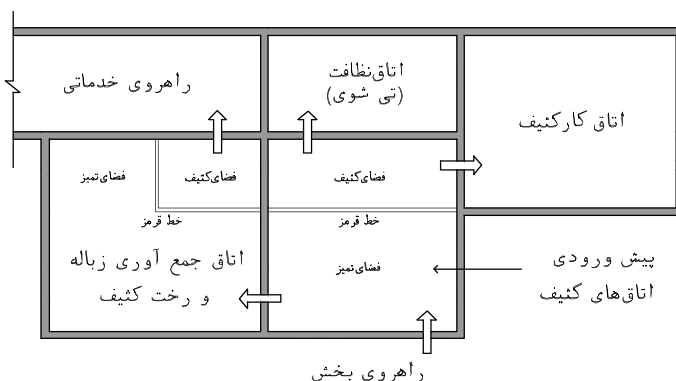
شکل ۲-۱۱- دسترسی از پیش‌ورودی اتاق‌های کثیف به اتاق جمع‌آوری زباله و رخت کثیف متصل به راهروی خدماتی
