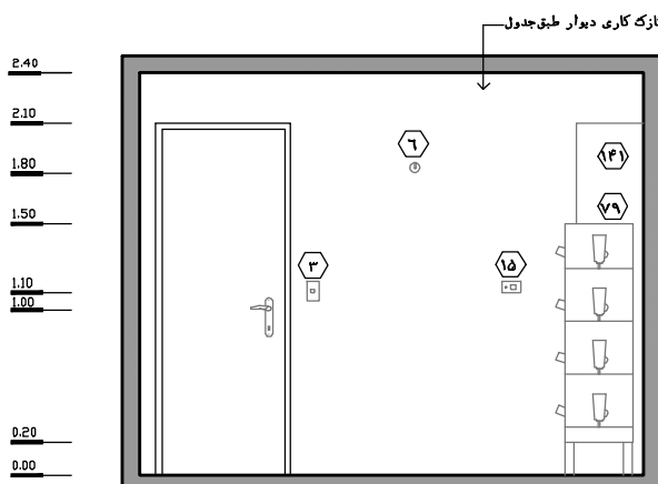
نقشه‌ی ۲-۹۶- نمای ۲ - مقیاس ۱:۵۰
