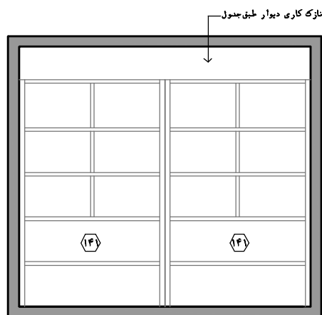
نقشه ۲-۱۱۸- نمای ۱ مقیاس ۱:۵۰
