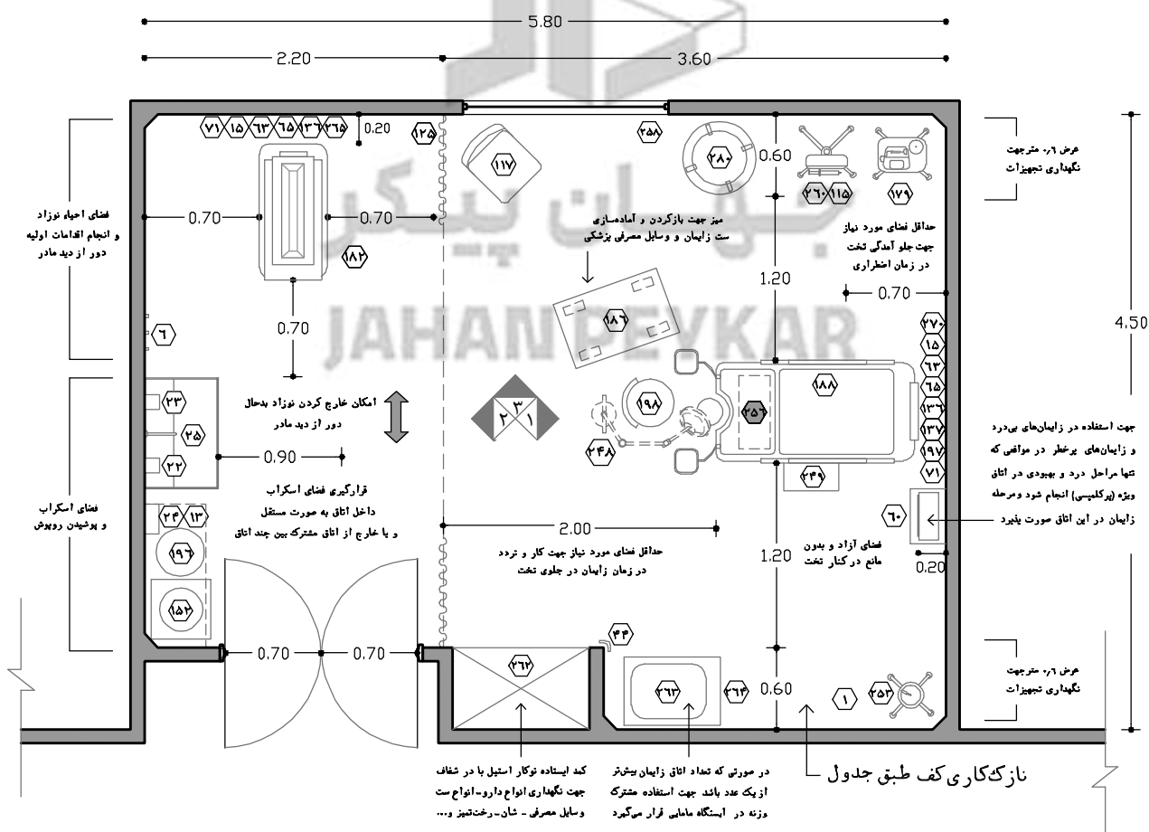
نقشه‌ی ۲-۴۷- پلان نمونه‌ی اتاق زایمان (برای ۴۰۰۰ زایمان سالانه) - مقیاس ۱:۵۰
