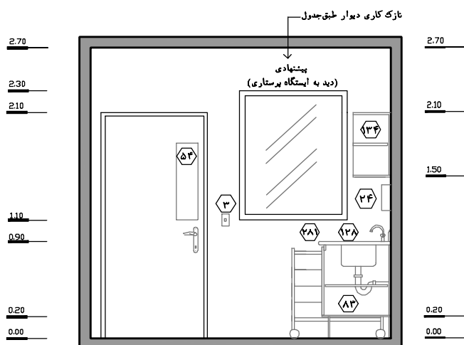
نقشه ۲-۷۵ - نمای ۱ - مقیاس ۱:۵۰
