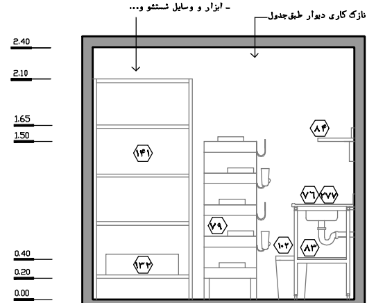
نقشه ۲-۹۷- نمای ۳ - مقیاس ۱:۵۰
