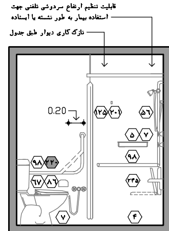
نقشه ۵-۴۵-نمای ۵ - مقیاس ۱:۵۰
