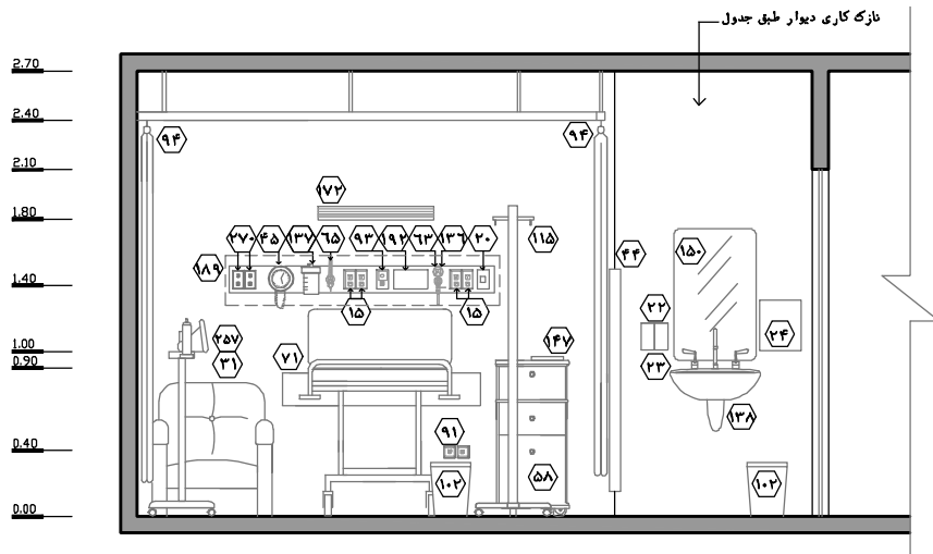
نقشه ۲-۴۱-نمای ۱ - مقیاس ۱:۵۰
