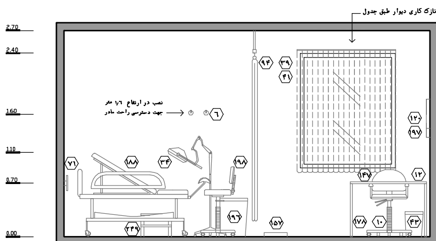
نقشه‌ی ۲-۱۷- نمای ۱- مقیاس ۱:۵۰
