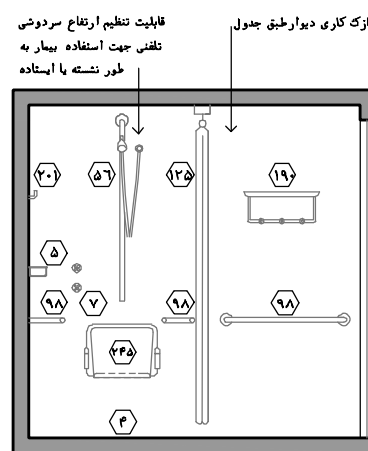
نقشه ۴-۴۴-نمای ۴ - مقیاس ۱:۵۰
