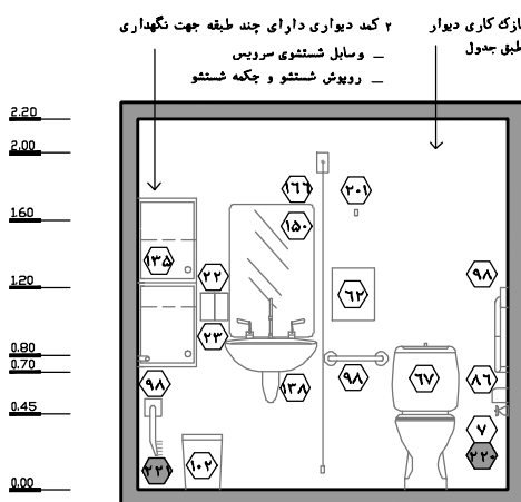
نقشه ۳-۴۳-نمای ۳ - مقیاس ۱:۵۰
