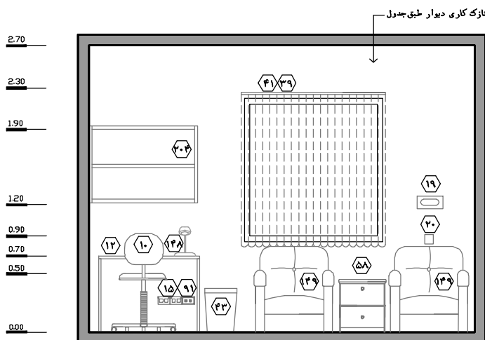
نقشه‌ی ۲-۸۶- نمای ۱ - مقیاس ۱:۵۰
