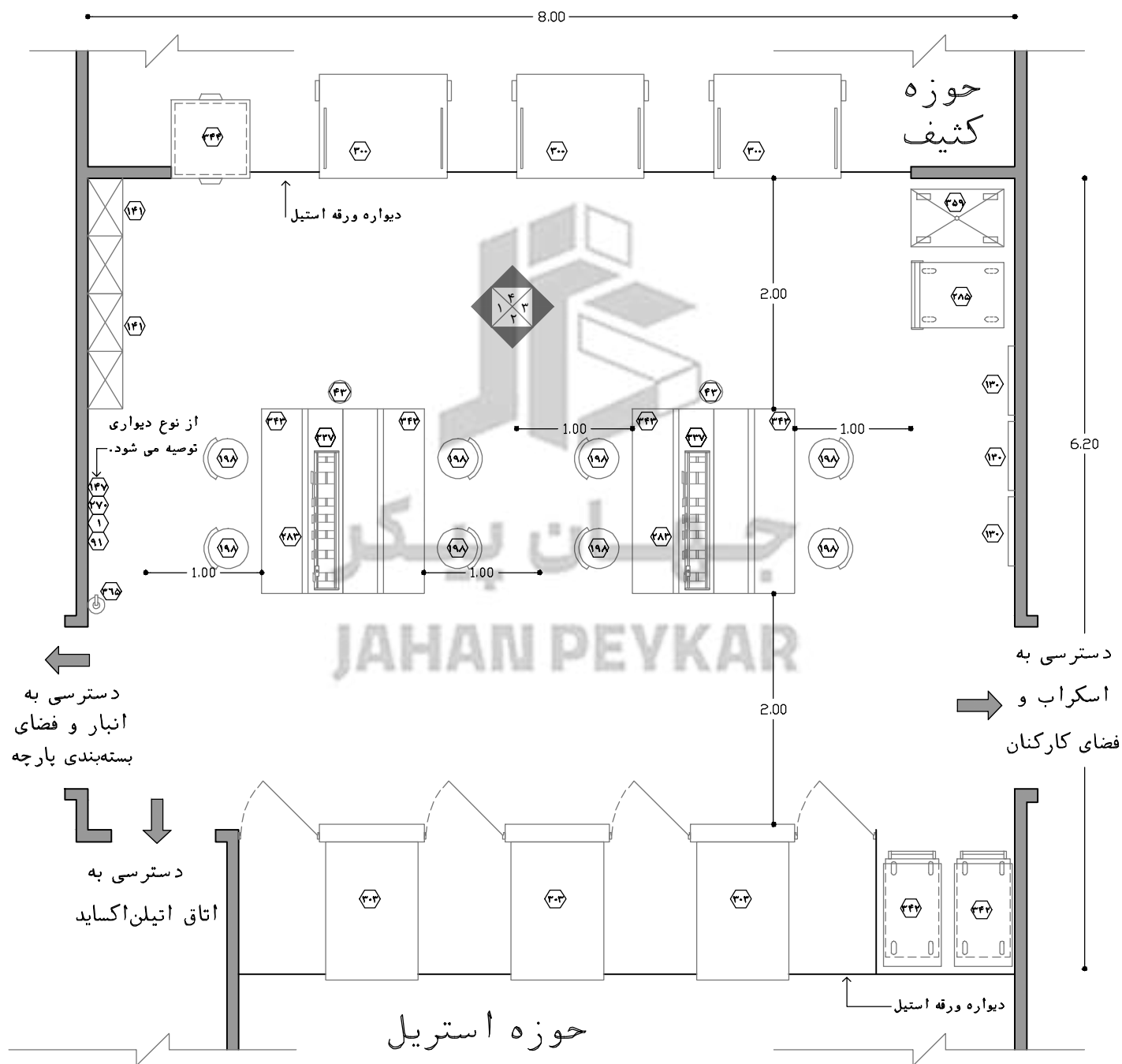
نقشه ۲-۳۱- پلان نمونه‌ی فضای آماده‌سازی و بسته‌بندی (حوزه تمیز) - مقیاس ۱:۵۰
