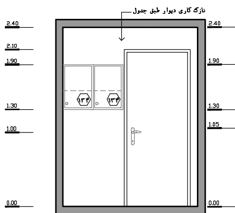
نقشه‌ی ۳-۲۰- نمای ۳ - مقیاس ۱:۵۰
