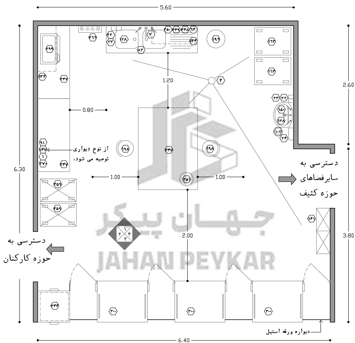
نقشه ی ۱۶-۲- پلان نمونه ی فضای شستشو و ضدعفونی (حوزه کثیف) - مقیاس ۱:۵۰
