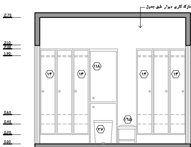
نقشه ۵-۲ - نمای ۴ - مقیاس ۱:۵۰
