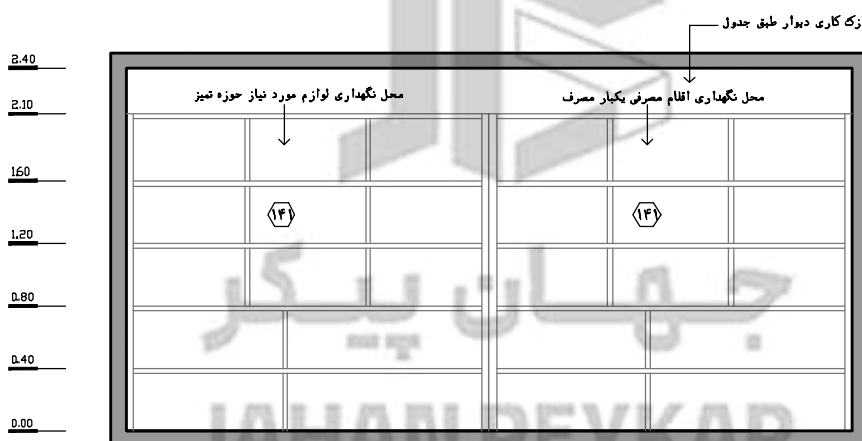
نقشه‌ی ۵۲-۲- نمای ۱ - مقیاس ۱:۵۰
