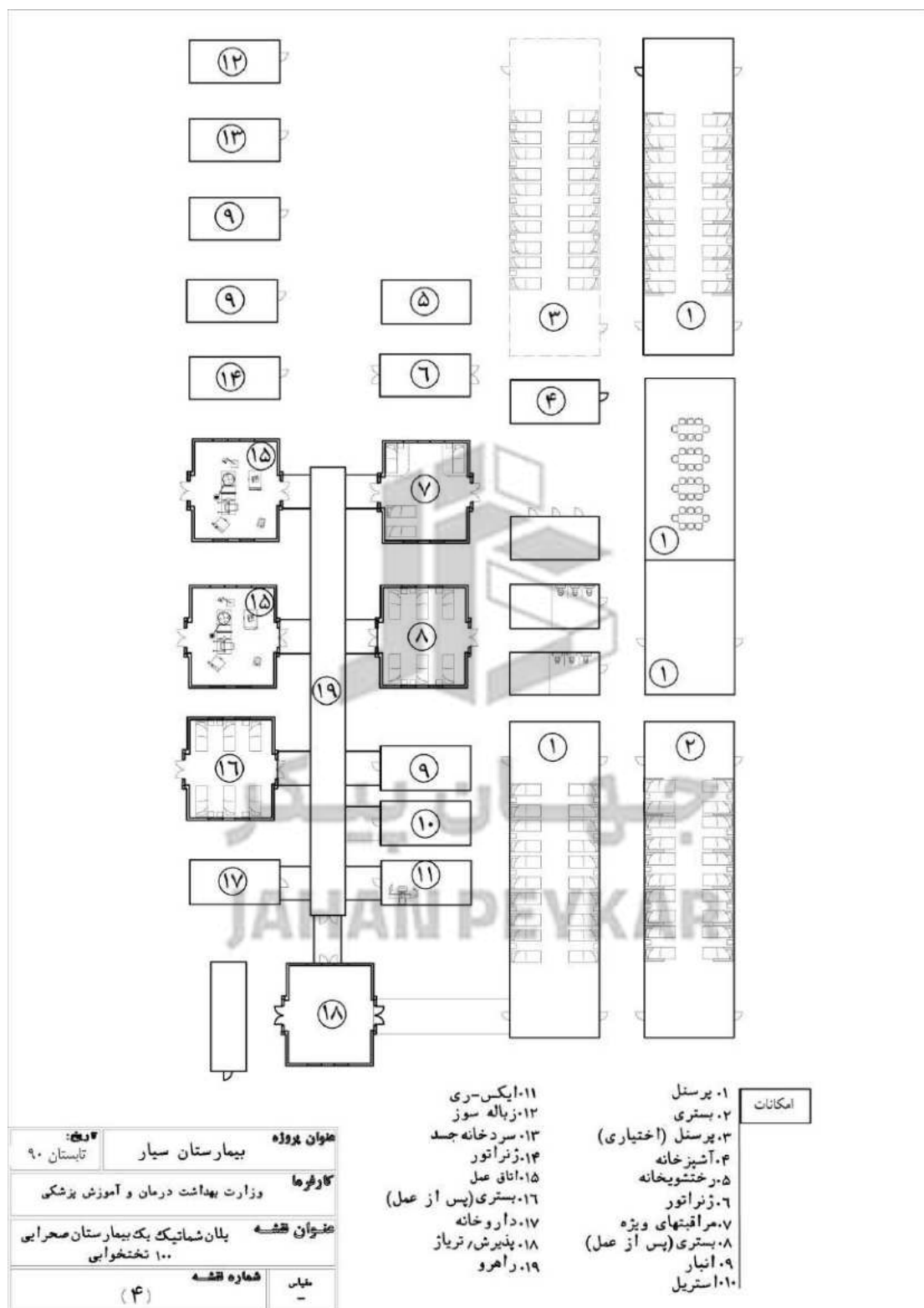
شکل ۱۶-۶ پلان شماتیک یک بیمارستان صحرائی ۱۰۰ تختخواهی
