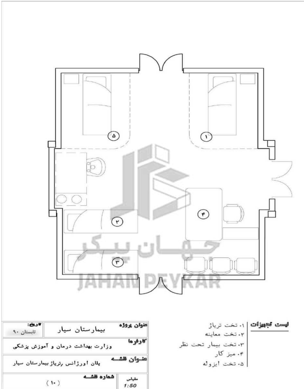
شکل ۶-۱ پلان اورژانس، تریاز بیمارستان سیار
